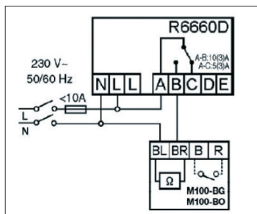
Verkabelung z.B. zum Thermoantrieb M100-BG oder M100-BO
